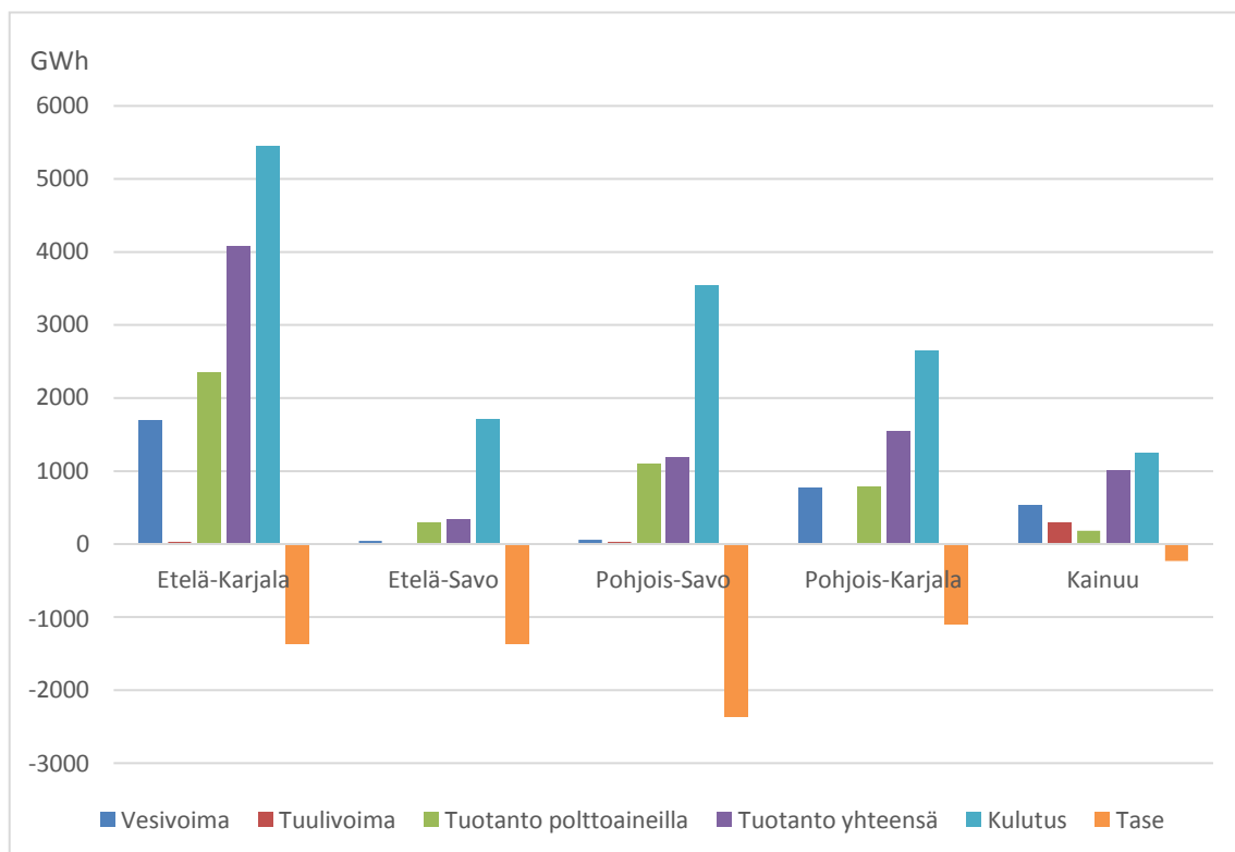
Kuva 7. Itä-Suomen maakuntien sähköntuotanto tuotantomuodoittain, kulutus, ja sähkötase 2018 (GWh)
